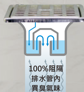
PKU531 泰晤士存水防臭 尺寸：9.5x9.5cm 面蓋： 7mm厚度 管徑：2"(A)
