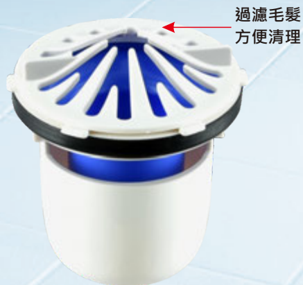
PK430 菊花型防臭小丸子 尺寸：9.3x9.3cm 面蓋：0.6mm 管徑：2"(O) 2"(A)
