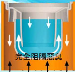
防臭水封結構
