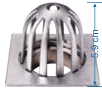
PD740S PD740SA (附網) 銅鍍鉻高腳落水頭 尺寸：9.3x9.3x5.9cm 口徑：2"
