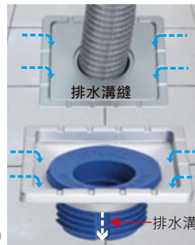
PK615B (厚管) 軟管塞頭 尺寸：6.7x6.7x3.2cm 口徑：2"x1¼"
