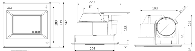
TV258 矩形面板 靜音換氣扇
